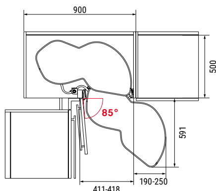
Primer: izvlači se udesno (levi ormarić – vrata širine 45 cm)
