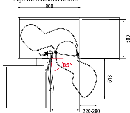
Primer: izvlači se udesno (levi ormarić – vrata širine 40 cm)
