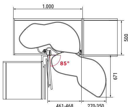
Primer: izvlači se udesno (levi ormarić – vrata širine 50 cm)
